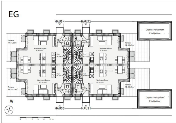
Grundriss Erdgeschoss
