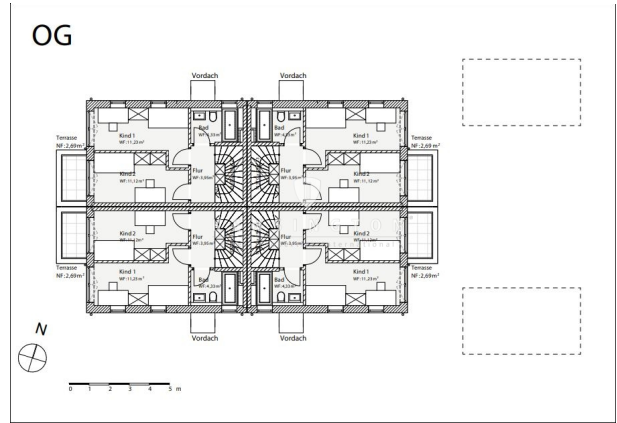
Grundriss Obergeschoss
