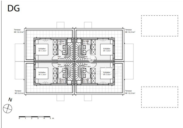
Grundriss Dachgeschoss
