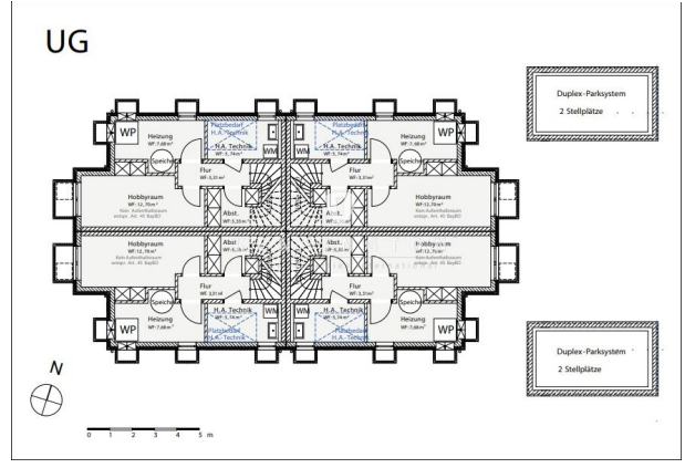
Grundriss Untergeschoss
