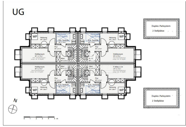
Grundriss Untergeschoss
