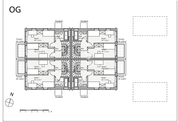
Grundriss Obergeschoss
