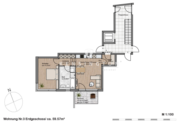
Wohnung Nr. 3
