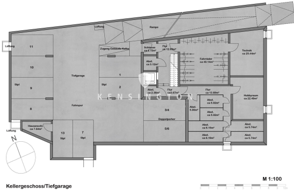
Kellergeschoss/Tiefgarage
