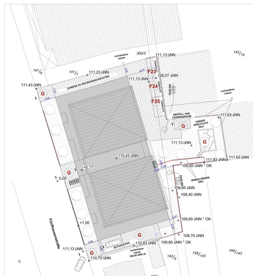
LAGEPLAN M=1:200
