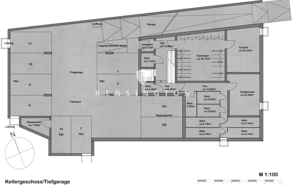
Kellergeschoss/Tiefgarage
