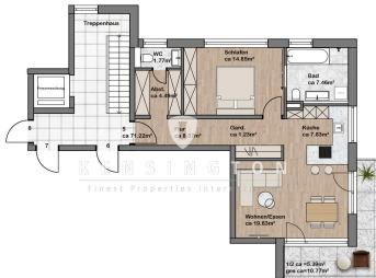
Wohnung Nr.5 Obergeschoss/ ca. 71,22m²
